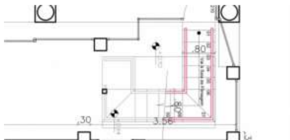
FIGURA 13: RECORTE DA PLANTA DA LOCALIZAÇÃO DA ESCADA QUE NECESSITA DO PATAMAR
